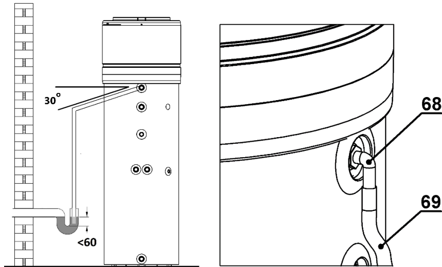
Fig. 9 - Exemplo de conexão do tubo de drenagem de condensação via sifão
