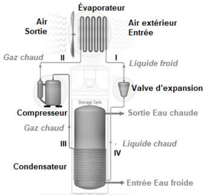
Fig.1 – Principe de fonctionnement ►
