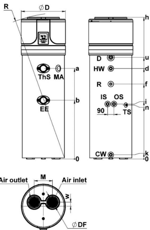
Fig. 7 – Dimensiones totales
