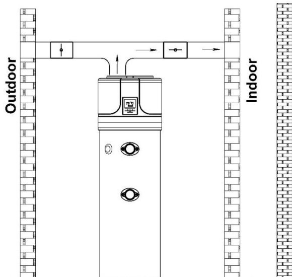
Fig. 6a – Ejemplo de instalación durante el verano
