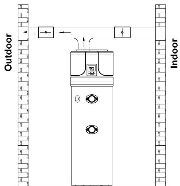
Fig. 6b Variante de instalação de inverno
