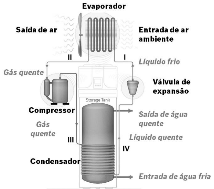
Figura 1 - Princípio de operação
