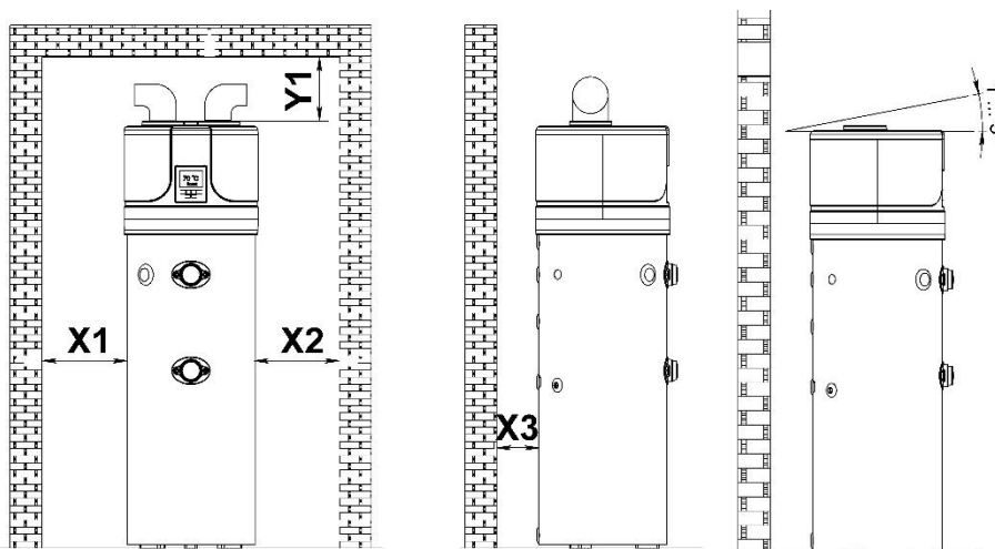
Fig. 4a - Espaço mínimo e instalação sem condutas de ventilação
