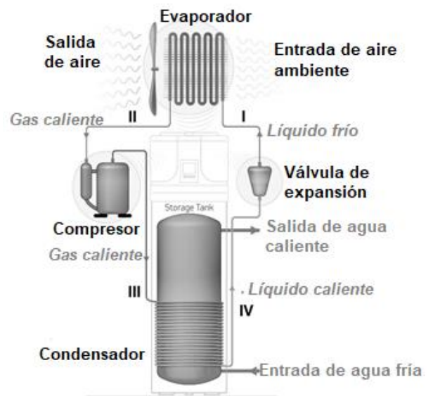
Fig.1 – Principio de operación ►
