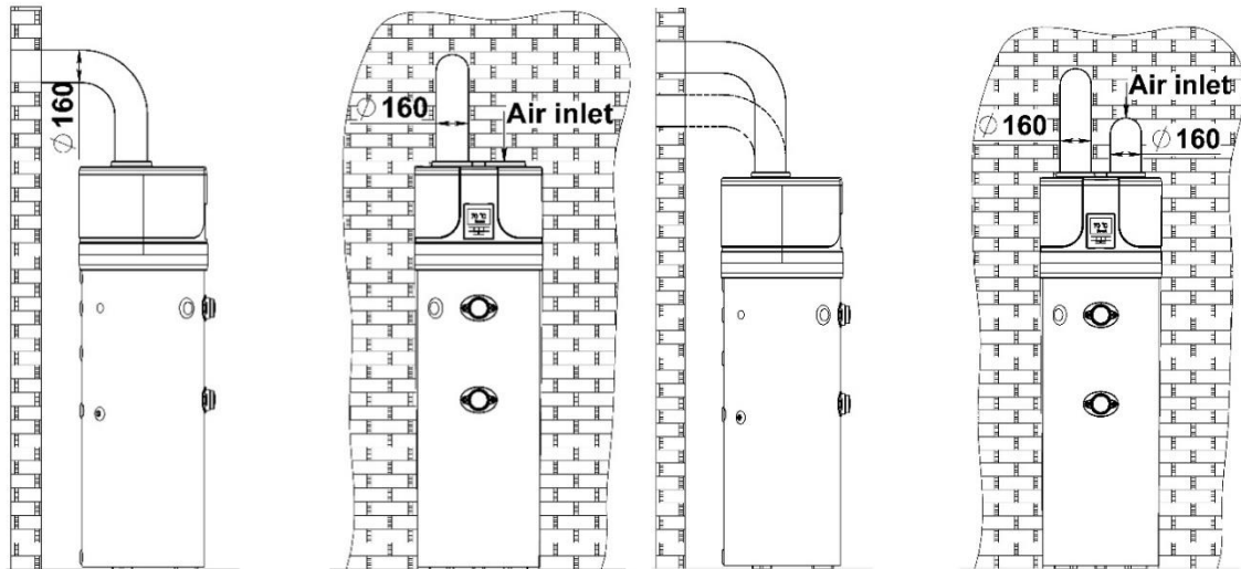
Fig. 5a - Exemplo de uma conduta de ventilação de exaustão Fig. 5b - Exemplo de conduta de ventilação dupla
