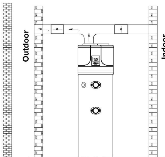
Fig. 6b Exemple d'installation en hiver
